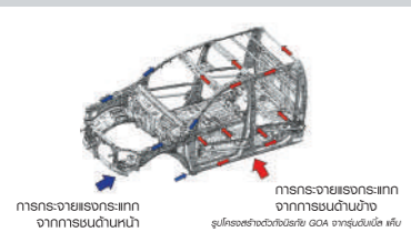
โครงสร้างตัวถังนิรภัย GOA ช่วยดูดซับแรงกระแทกและกระจายแรงกระแทก
